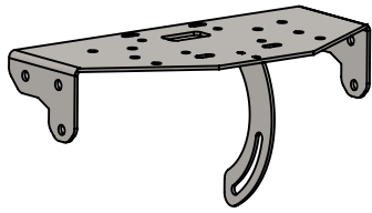
DİREKSİYON MONTAJ TABLASI
